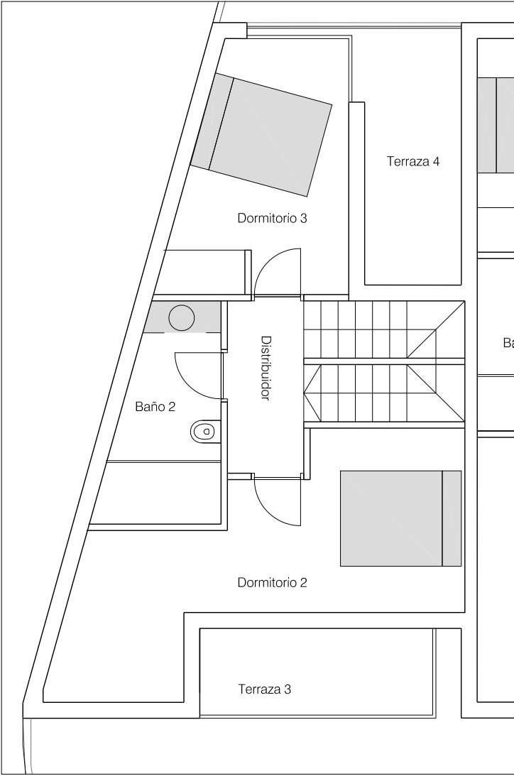
PLANTA SEGUNDA
