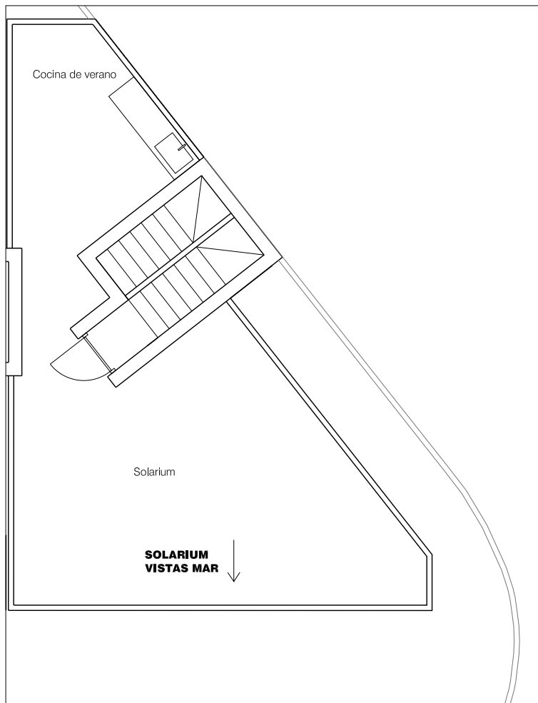
PLANTA SOLARIUM
