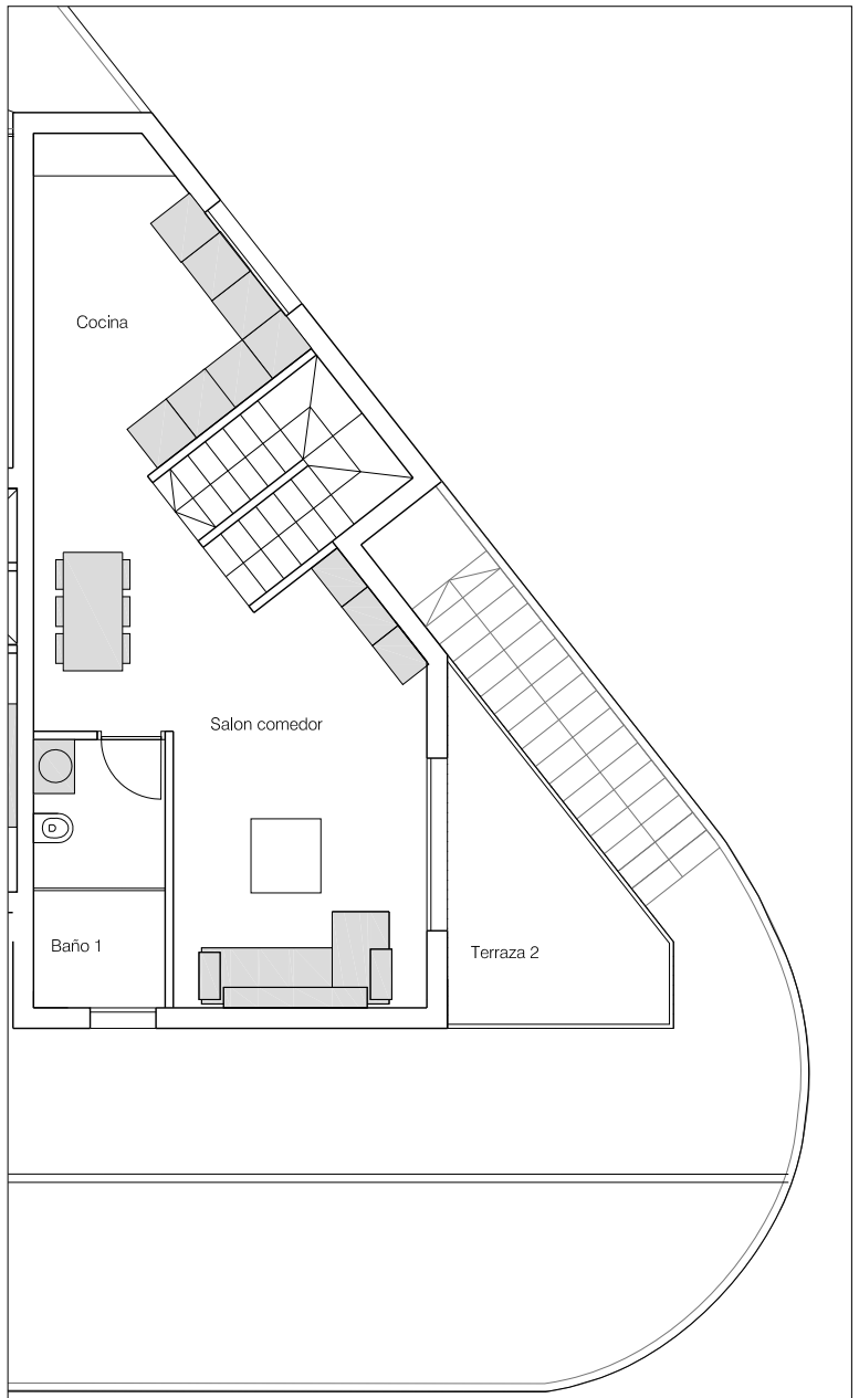
PLANTA SEGUNDA
