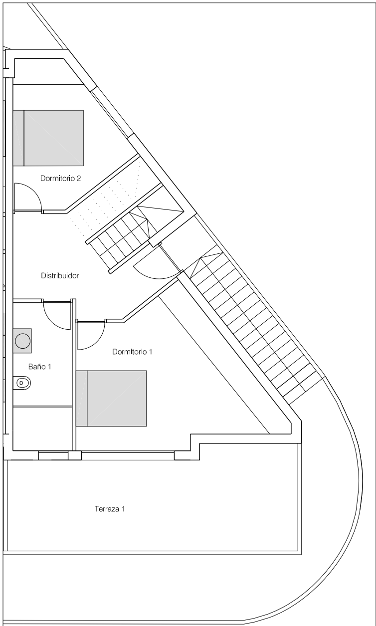
PLANTA PRIMERA
